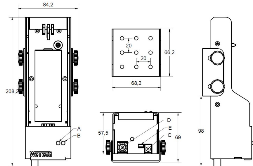
Schemazeichnung WTC623USB
